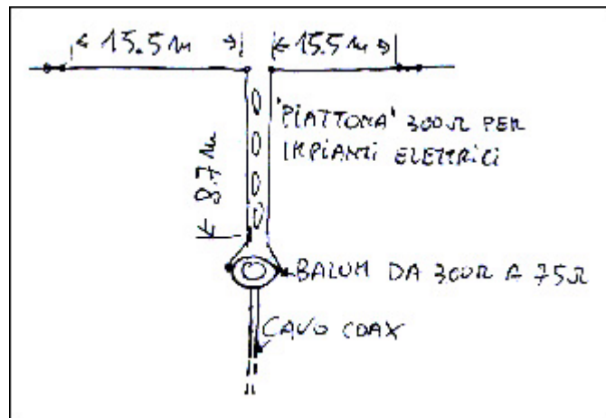
Schema pratico antenna G5RV.
